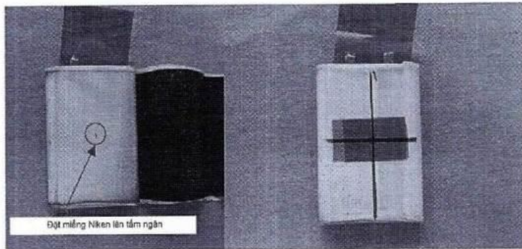
Cuộn điện cực và tấm ngăn lại, dán hai lớp băng polyamid tại vị trí miếng Niken
