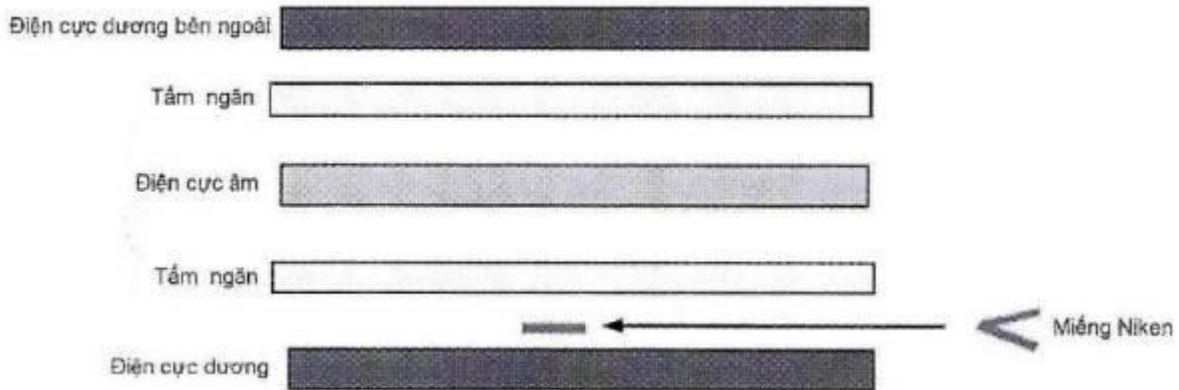
Hình A.8 - Vị trí của miếng Niken khi không thể đặt trong vùng quy định
