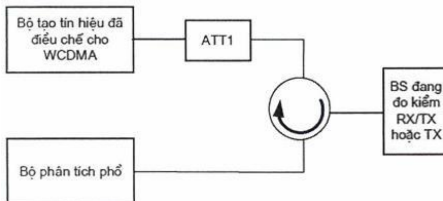
Hình D.3 - Sơ đồ đo công suất ra cực đại của trạm gốc
