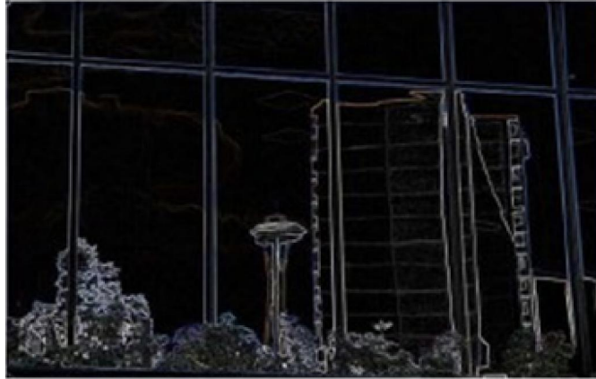
Sobel
