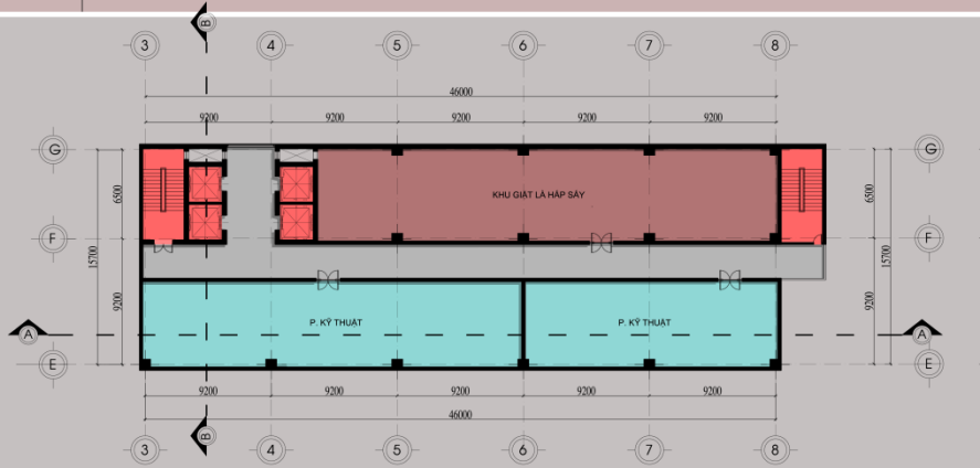
MẶT BẰNG TẦNG KỸ THUẬT TỶ LỆ 1:100
