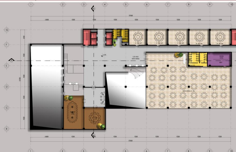
MẶT BẰNG TẦNG 2 TỶ LỆ 1:100
